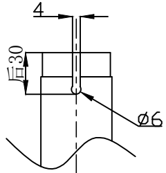
座管剖沟 (2:1)
