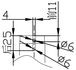
座管剖沟 (2:1)
