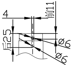
座管剖沟 (2:1)
