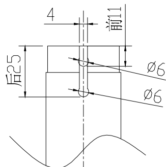
座管剖沟 (2:1)
