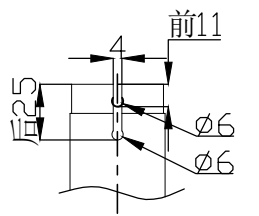
座管剖沟 (2:1)
